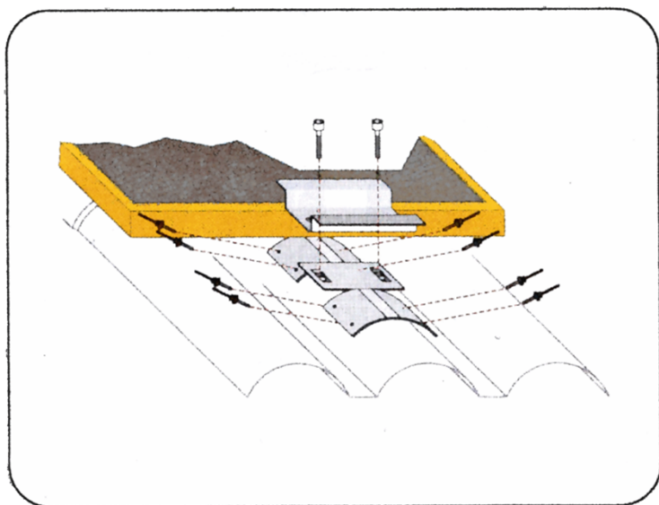
Esempio di fissaggio supporto intermedio con rivetti stagni su Tegomont standard
