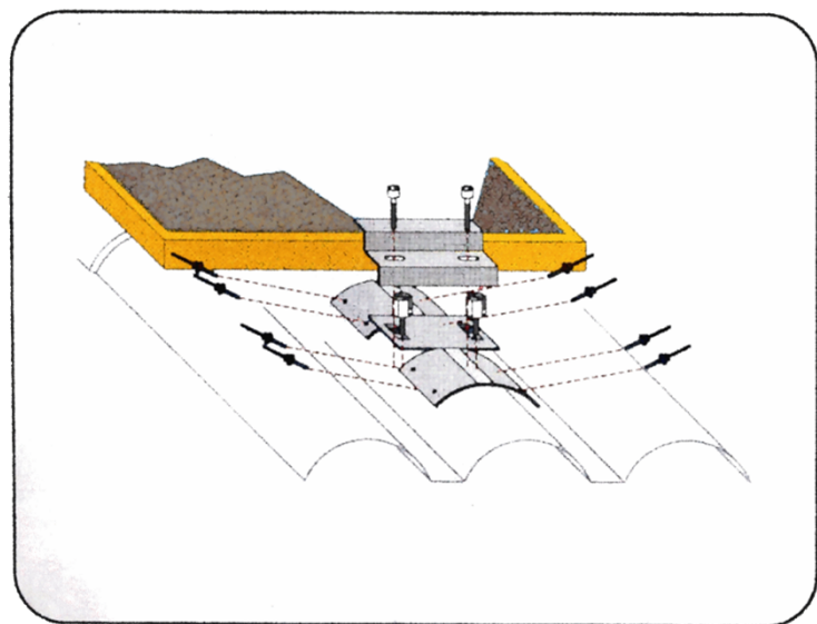
Esempio di fissaggio supporto terminale con rivetti stagni su Tegomont standard
